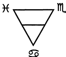
Группа 4 - вода
