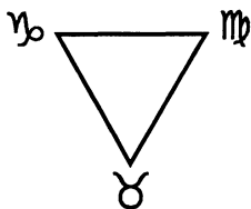
Группа 2 - земля
