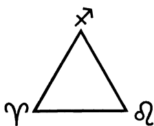
Группа 1 - огонь
