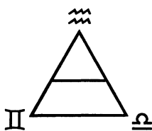
Группа 3 - воздух
