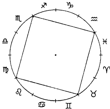
Рис. 7 Мутабельный крест
