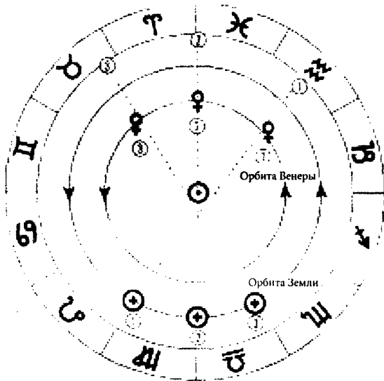
Ближние планеты в директном движении (вперед)
