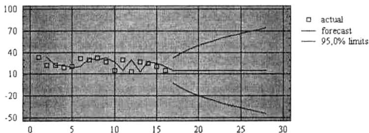
Табл.3. Прогноз по стохастической модели
