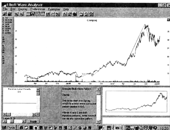
Табл. 8. Анализ волн Эллиотта [программа Bliott Wave Analyser]
