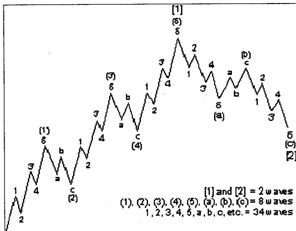
Табл. 7. Волна Эллиотта второго уровня
